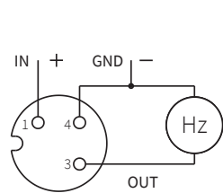
Frequenz Ausgang ungefiltert
