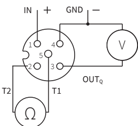
Spannung Ausgang mit Temperatur- messung PT1000
