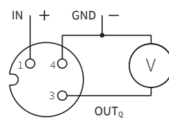
Spannung Ausgang
