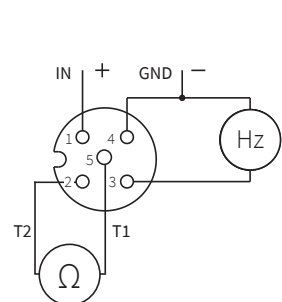
Frequenz Ausgang mit Temperaturmessung PT1000
